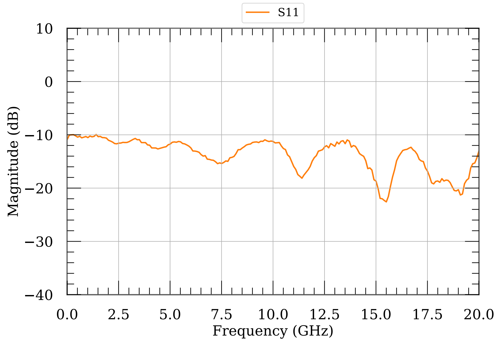
LNA S-params module059
